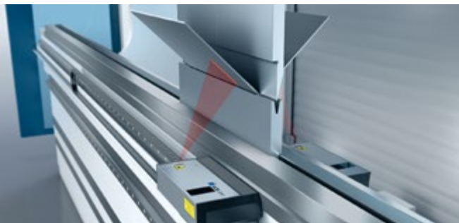
Präzise Winkel durch Lasermessung: ACB Laser.
