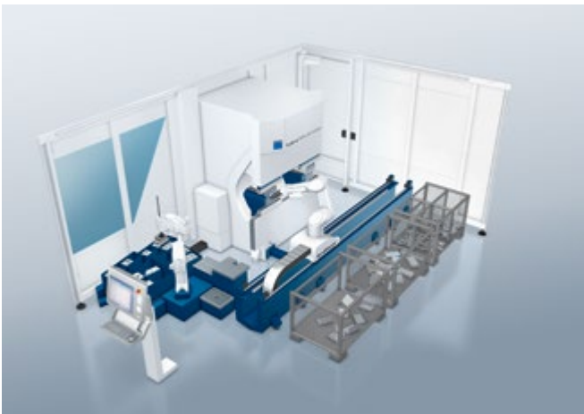
TruBend Cell 7000 mit BendMaster (15) und LoadMaster.
