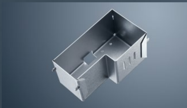
Je nach Maschine biegen Sie Schachtelhöhen bis zu 518 mm.
